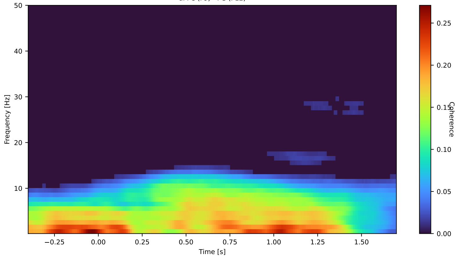
dPFC (F9) - PG (P12)
